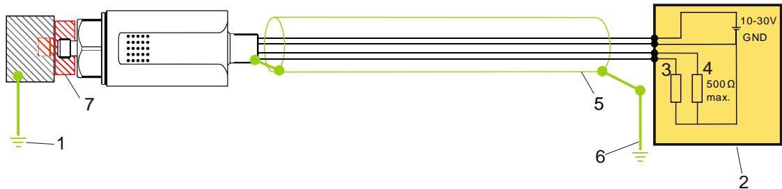
Рис. 11: Альтернативная концепция заземления
