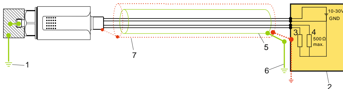
Рис. 10: Стандартная концепция заземления
